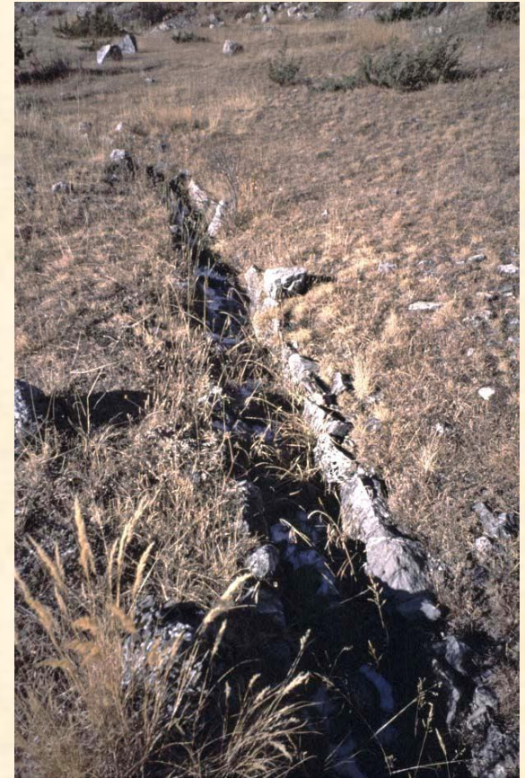
Canal en lauzes (Ceillac)
